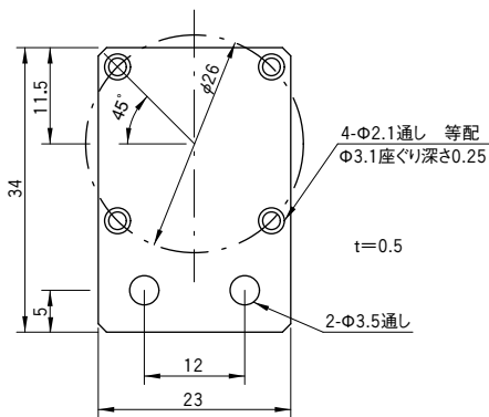
取付フランジ(付属品)
