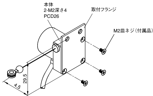
取付フランジ(付属品)
