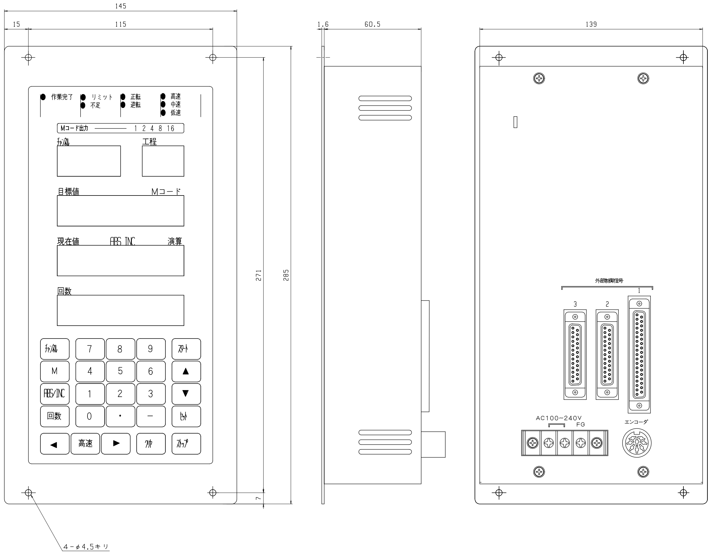
MPR-11 外形寸法図
